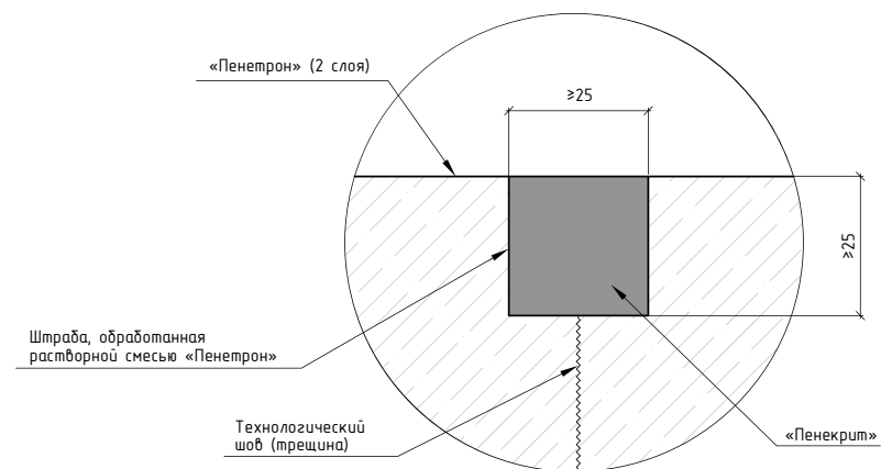
Рисунок 8.3 — Схема гидроизоляции шва бетонирования
