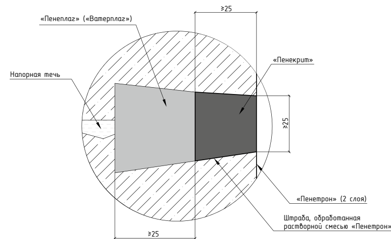
Рисунок 8.5 — Схема ликвидации течей
